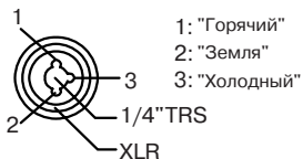
Симметричный джек
